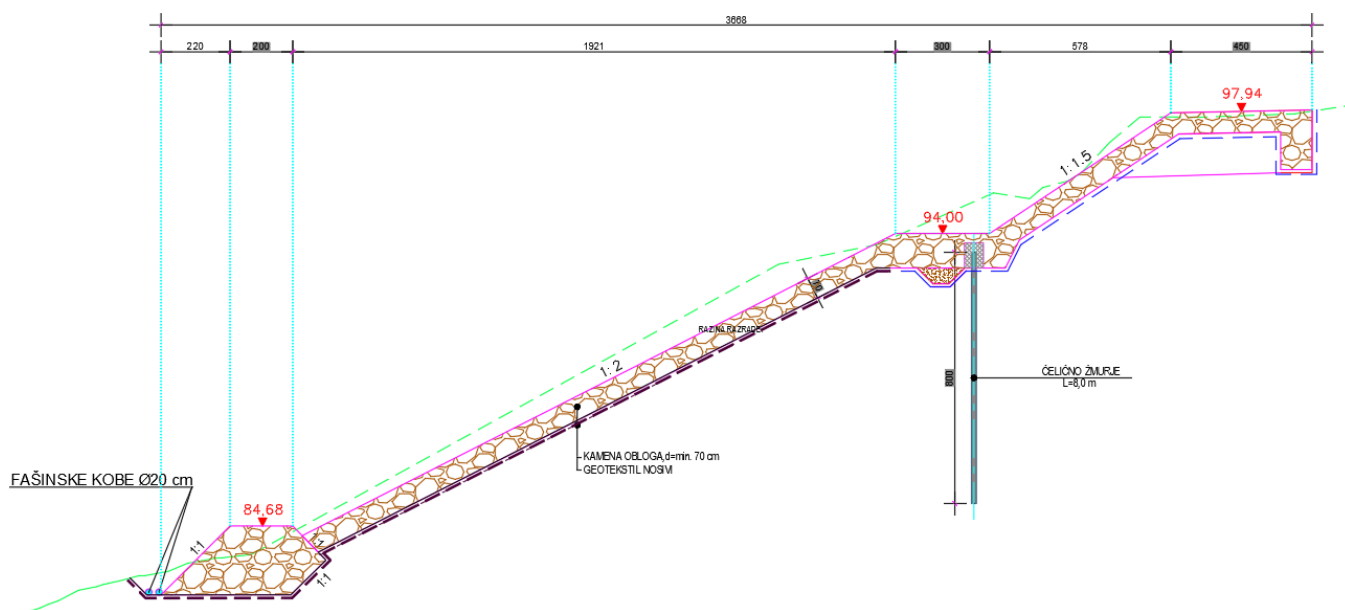
KARAKTERISTIČNI POPREČNI PRESJEK_Tip-B_P-7 0+060,00
