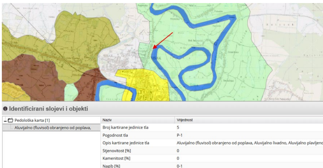
Slika 3-13: Pedološka karta u području zahvata (Izvor: https://envi.azo.hr/?topic=3 )
