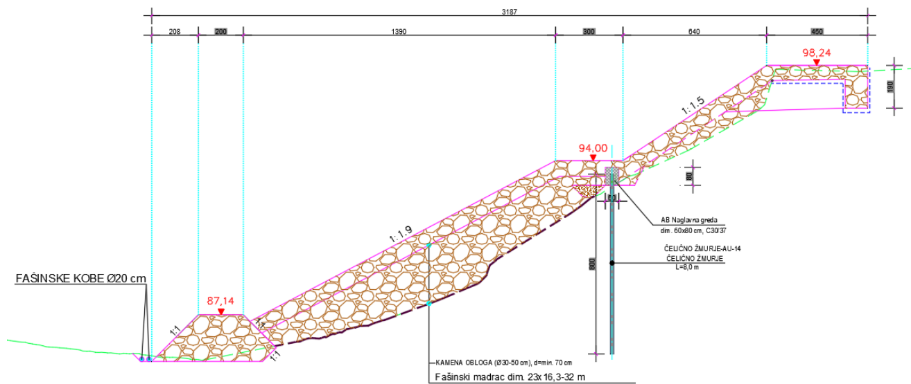
Slika 2-3: Prikaz karakterističnih poprečnih profila.
