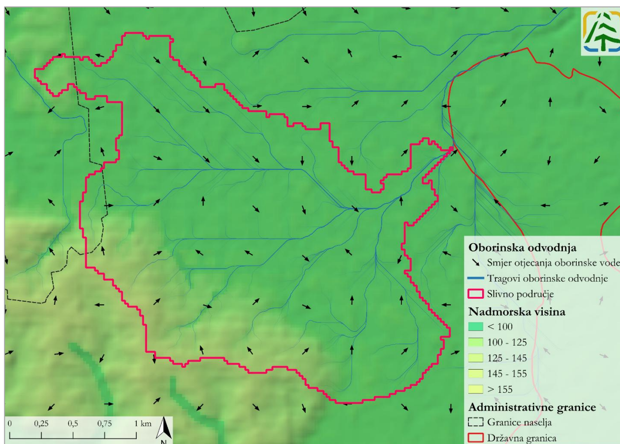
Slika 5.7 Smjer otjecanja oborinske odvodnje (Izvor: Geoportal DGU)
