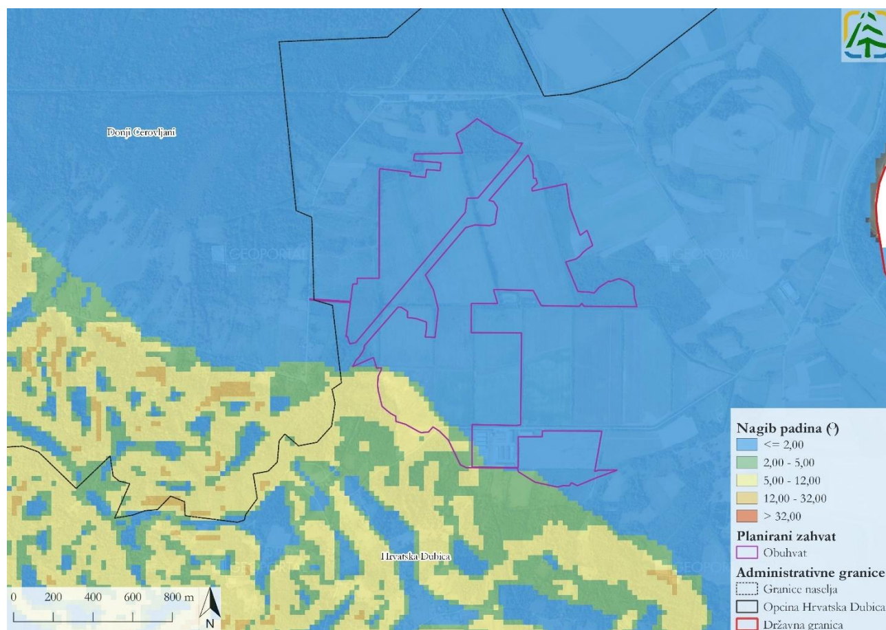
Slika 4.39 Nagib padina na širem području planiranog zahvata (Izvor: IGU, 1968, Idejno rješenje i Geoportal DGU)
