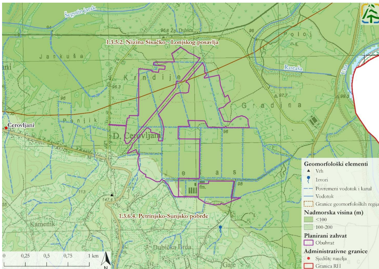
Slika 4.34 Elementi georaznolikosti i nadmorska visina (m) na širem području planiranog zahvata (Izvor: Idejno rješenje i TK25 – Geoportal DGU)
