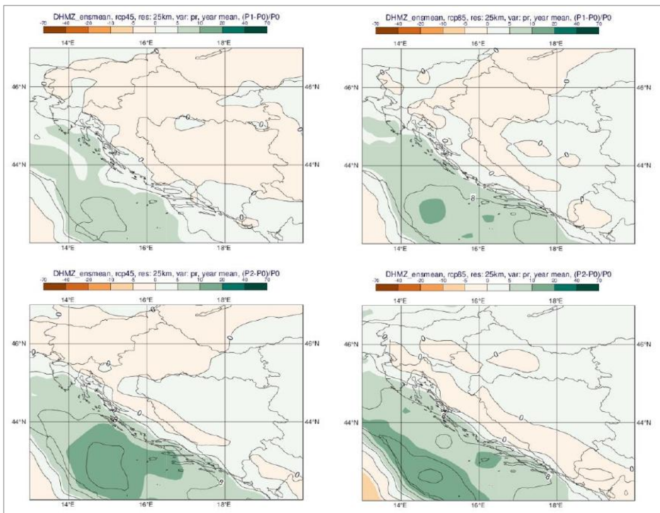
Slika 4.28 Promjena srednje godišnje ukupne količine oborine (%) u odnosu na referentno razdoblje 1971.-2000. u srednjaku ansambla iz četiri integracije RegCM modelom na rezoluciji 12,5 km. Gore: za razdoblje 2011.- 2040.; dolje: za razdoblje 2041.-2070.; lijevo: scenarij RCP4.5; desno: scenarij RCP8.5 (Izvor: Rezultati klimatskog modeliranja)
