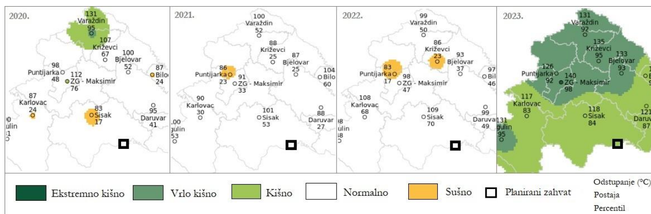
Slika 4.25 Odstupanje srednje količine oborine u razdoblju 2020. – 2023. godine na širem području planiranog zahvata (Izvor: DHMZ)
