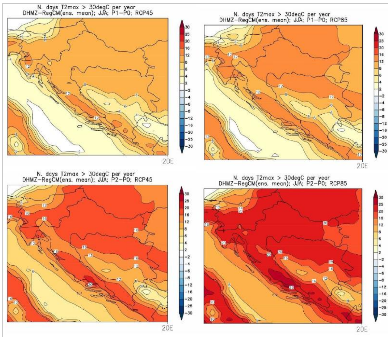
Slika 4.27 Promjena srednjeg broja vrućih dana u odnosu na referentno razdoblje 1971.- 2000. u srednjaku ansambla iz četiri integracije RegCM modelom na rezoluciji 12,5 km. Gore: za razdoblje 2011.-2040; dolje: za razdoblje 2041.-2070.; lijevo: scenarij RCP4.5; desno: scenarij RCP8.5. Sezona: ljeto (Izvor: Rezultati klimatskog modeliranja)
