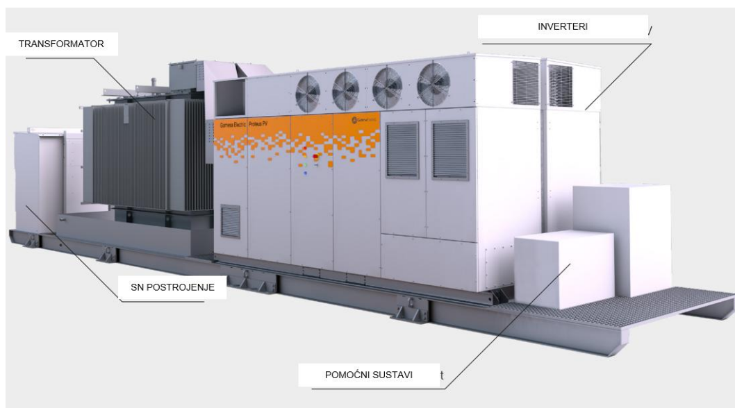
Slika 2.7 Interna TS (Izvor: Idejno rješenje)
