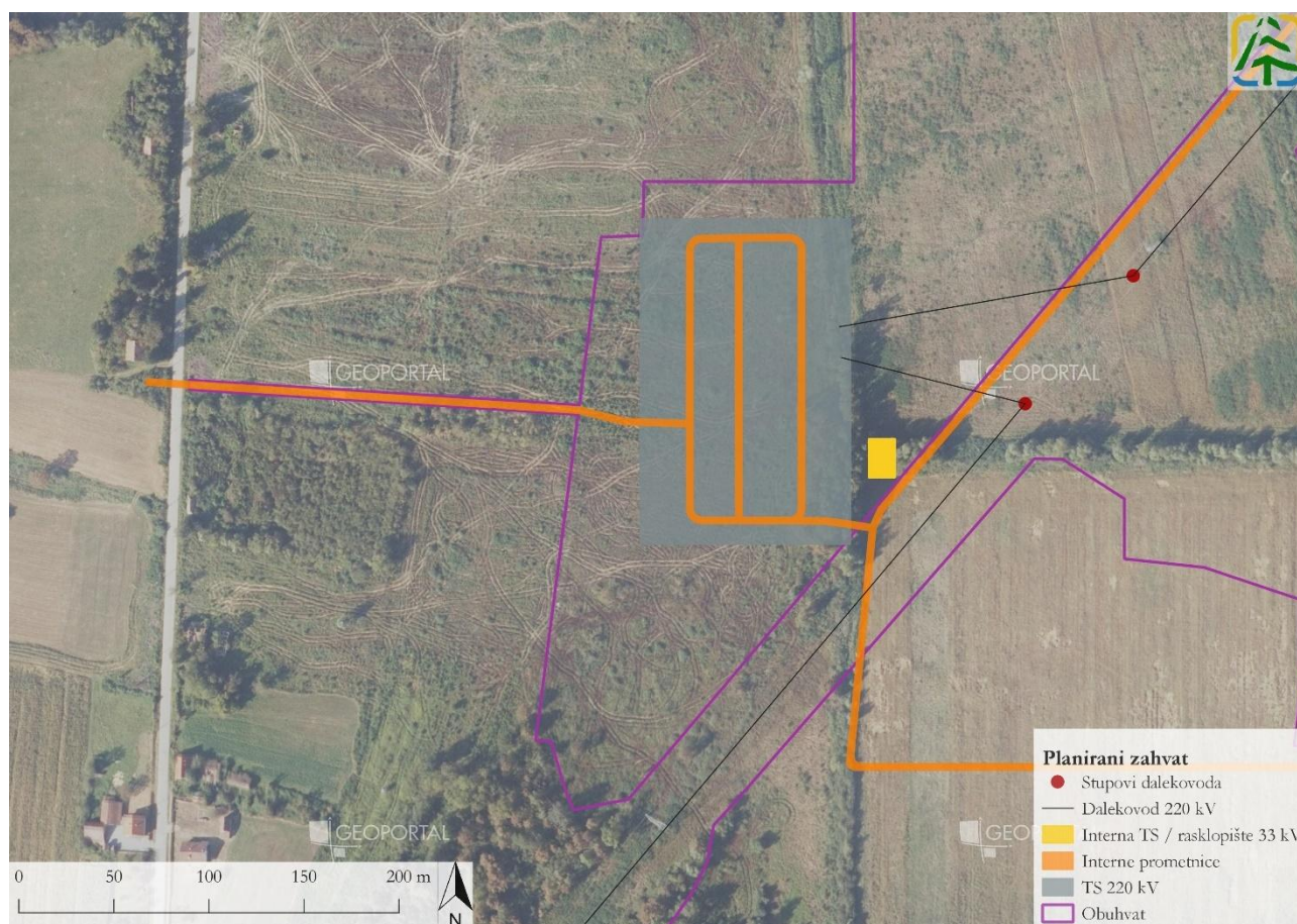
Slika 2.8 Lokacija planirane trafostanice za potrebe SE Hrvatska Dubica
