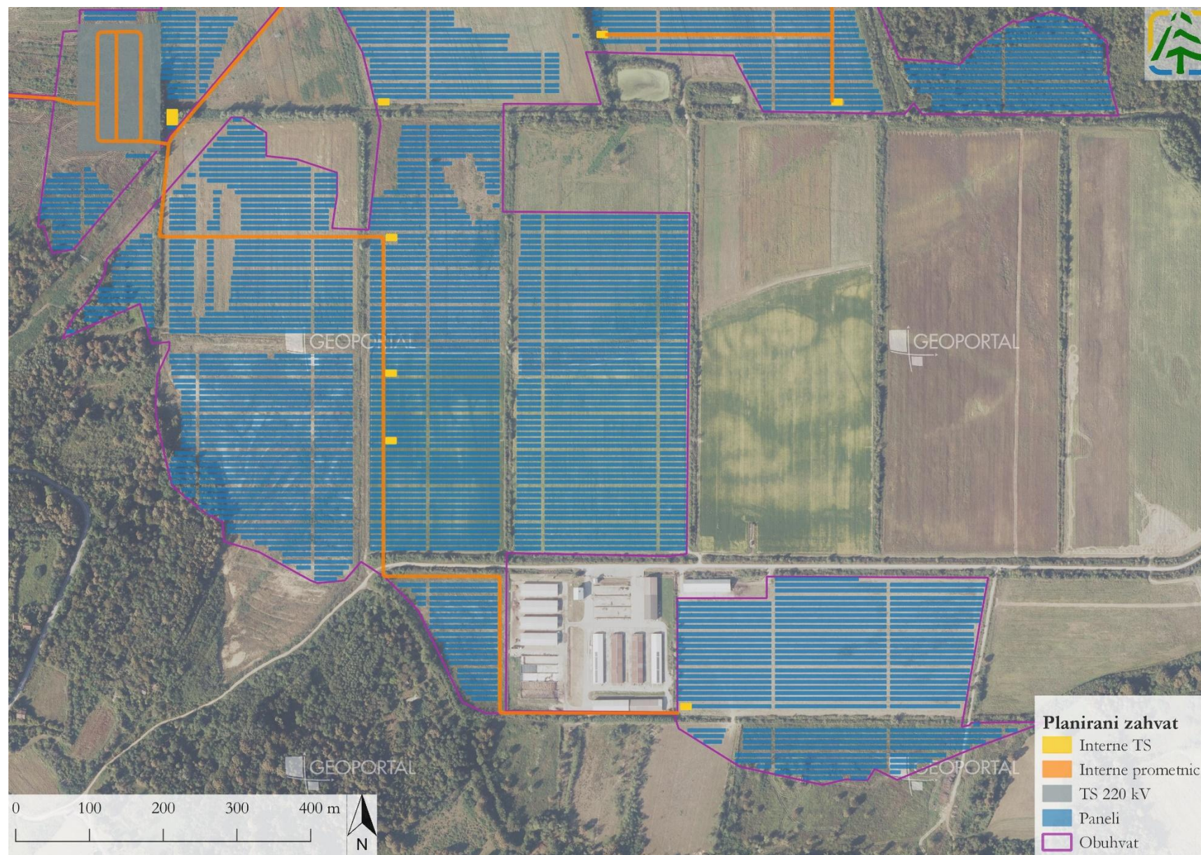
Slika 2.3 Elementi planiranog zahvata – južni dio (Izvor: Idejno rješenje, Geoportal DGU)
