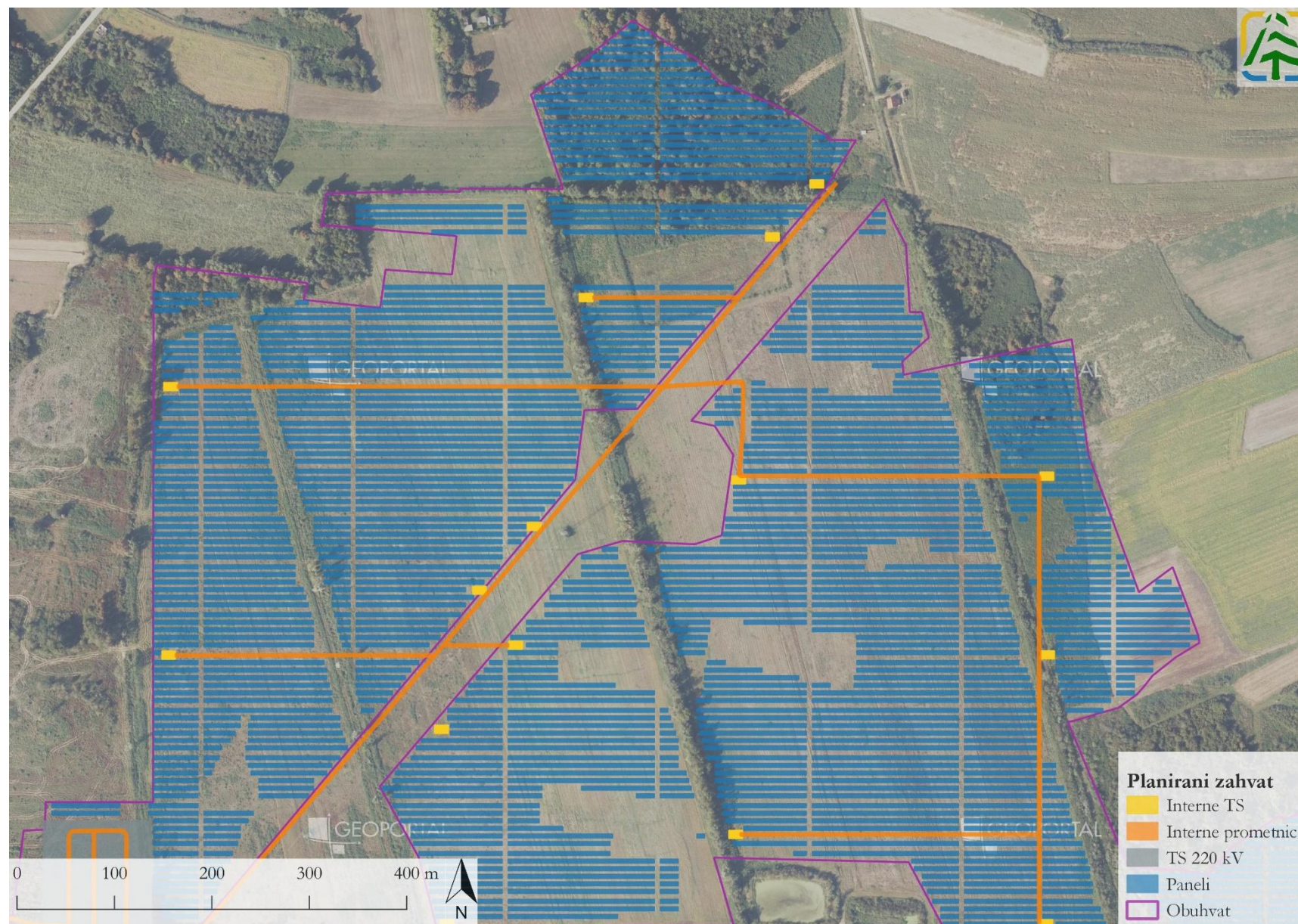
Slika 2.4 Elementi planiranog zahvata – sjeverni dio (Izvor: Idejno rješenje, Geoportal DGU)
