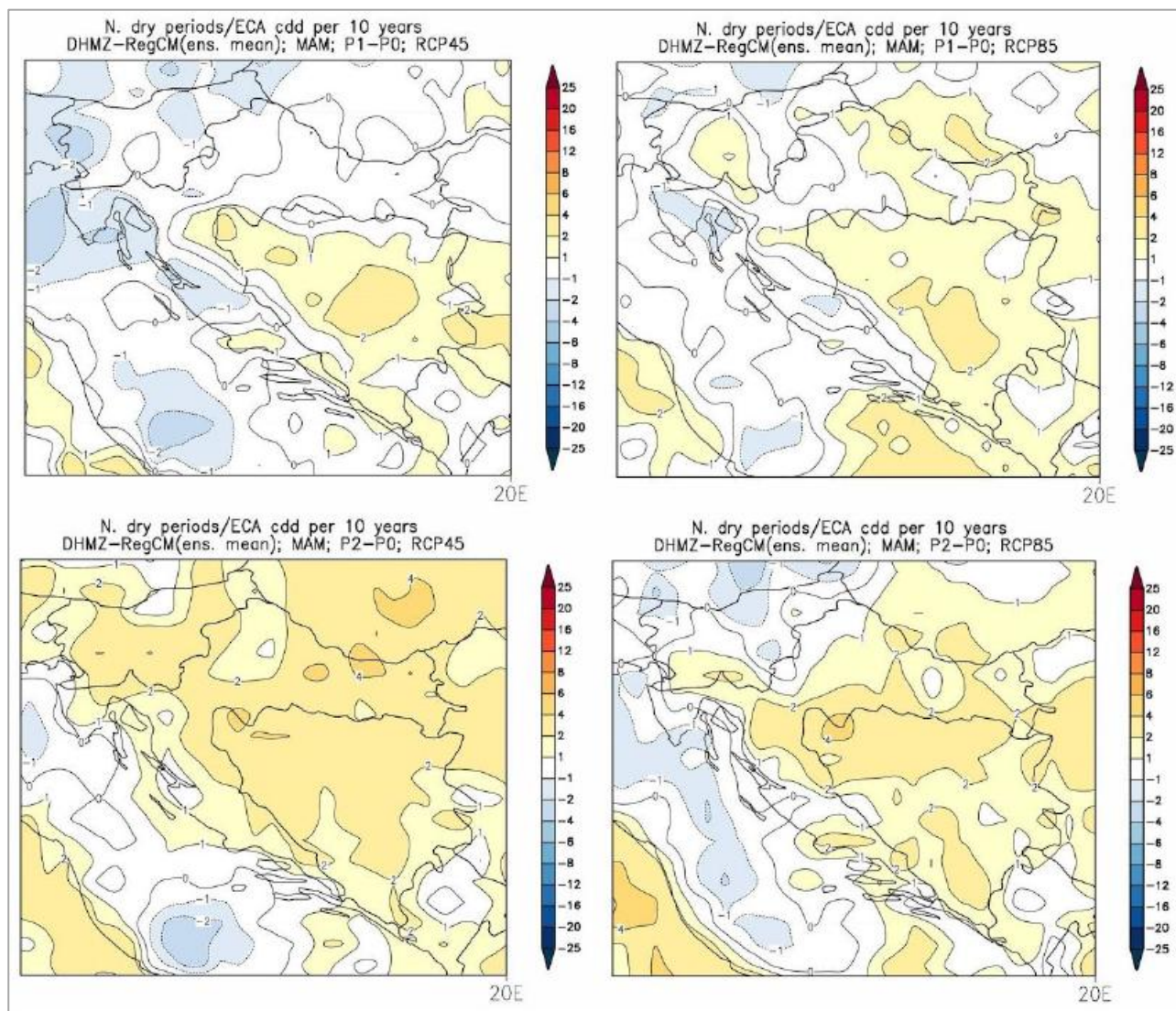
Slika 4.30 Promjena broja sušnih razdoblja u odnosu na referentno razdoblje 1971.-2000. u srednjaku ansambla iz četiri integracije RegCM modelom na rezoluciji 12,5 km. Gore: za razdoblje 2011.-2040.; dolje: za razdoblje 2041.-2070.; lijevo: scenarij RCP4.5; desno: scenarij RCP8.5 (Izvor: Rezultati klimatskog modeliranja)
