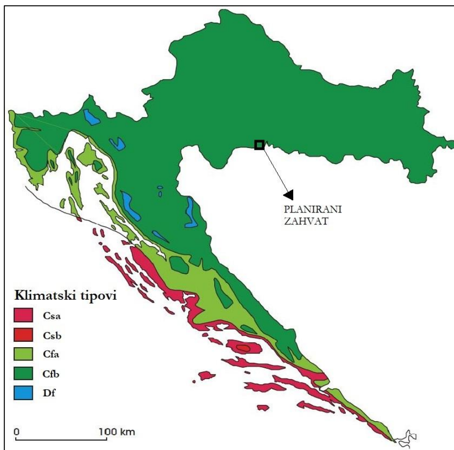
Slika 4.21 Geografska raspodjela klimatskih tipova po W. Köppenu u Hrvatskoj u standardnom razdoblju od 1961. do 1990. (Izvor: Šegota i Filipčić, 2003)
