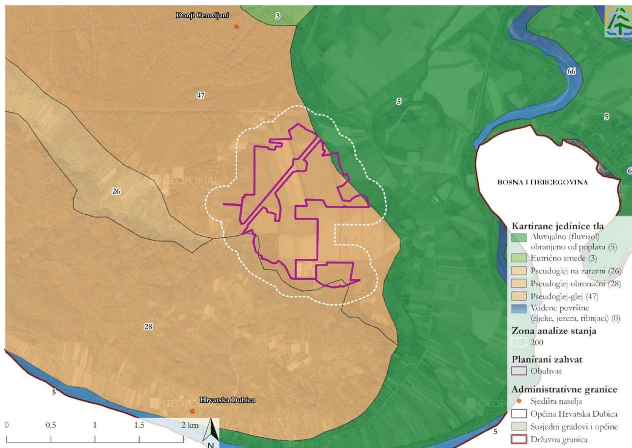
Slika 4.35 Kartirane jedinice tla na području zone analize stanja planiranog zahvata (Izvor: Namjenska pedološka karta RH, Idejno rješenje i Geoportal DGU)
