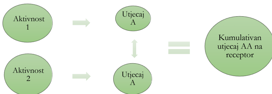
Slika 5.8 Ilustracija koncepta kumulativnih utjecaja planiranog zahvata
