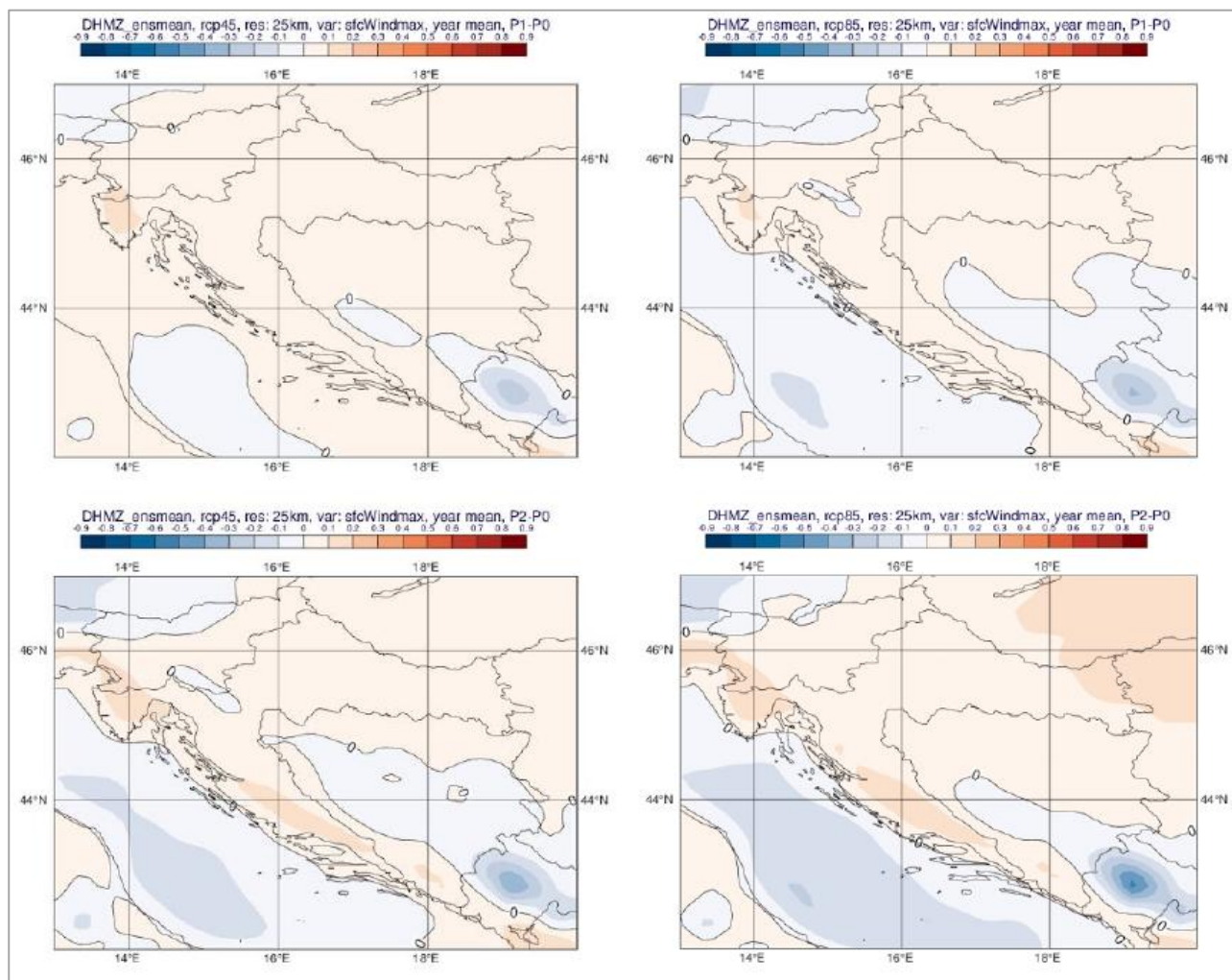
Slika 4.29 Promjena srednje godišnje maksimalne brzine vjetra na 10 m (m/s) u odnosu na referentno razdoblje 1971.-2000. u srednjaku ansambla iz četiri integracije RegCM modelom na rezoluciji 12,5 km. Gore: za razdoblje 2011.-2040.; dolje: za razdoblje 2041.-2070.; lijevo: scenarij RCP4.5; desno: scenarij RCP8.5 (Izvor: Rezultati klimatskog modeliranja)
