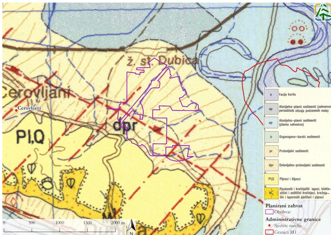
Slika 4.31 Položaj planiranog zahvata na OGK SFRJ 1:100 000, list Kostajnica (Izvor: Idejno rješenje, Jovanović i Magaš, 1986)
