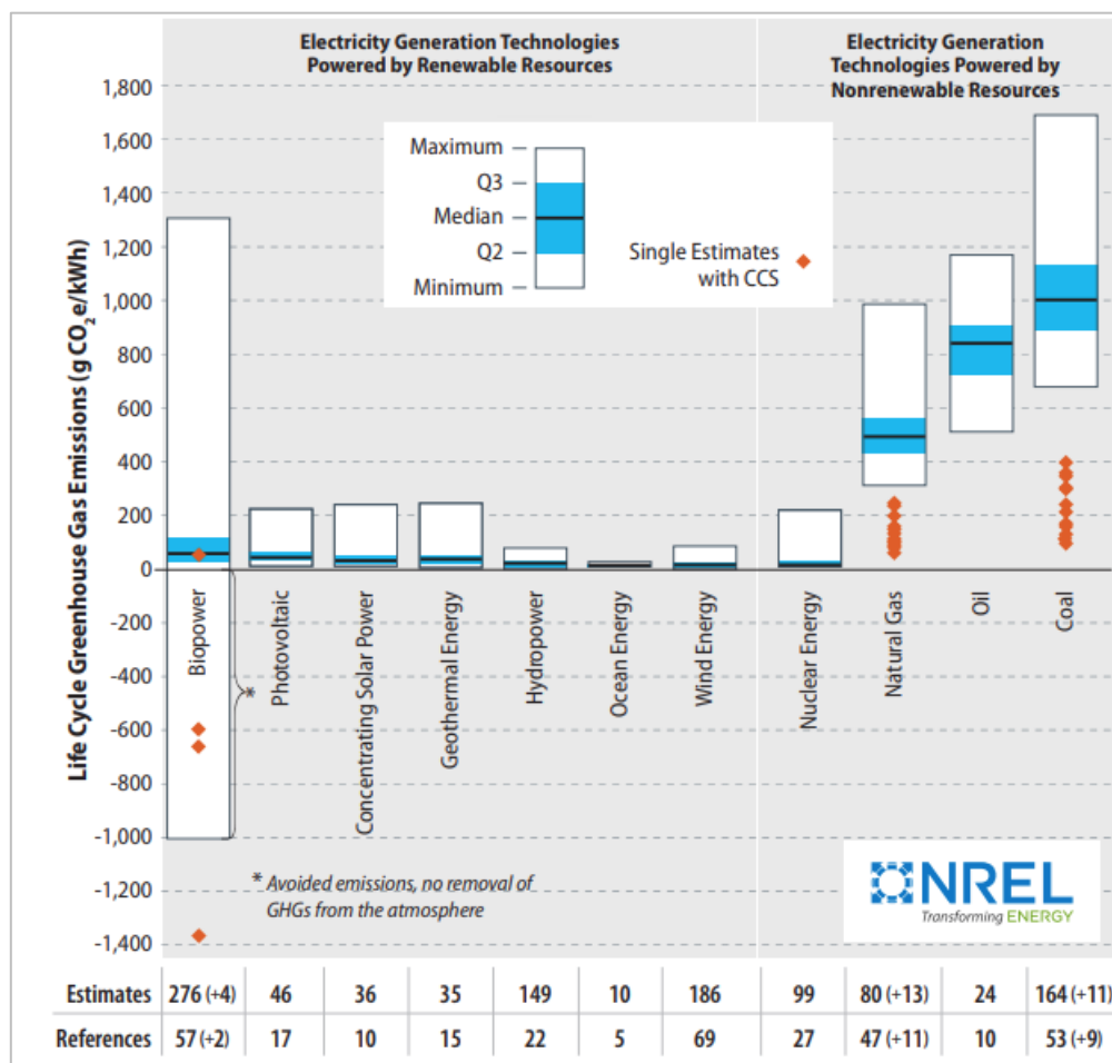
Slika 5.1 Emisije stakleničkih plinova za različite sustave proizvodnje električne energije tijekom njihovog životnog ciklusa (Izvor: National Renewable Energy Laboratory, 2021)
