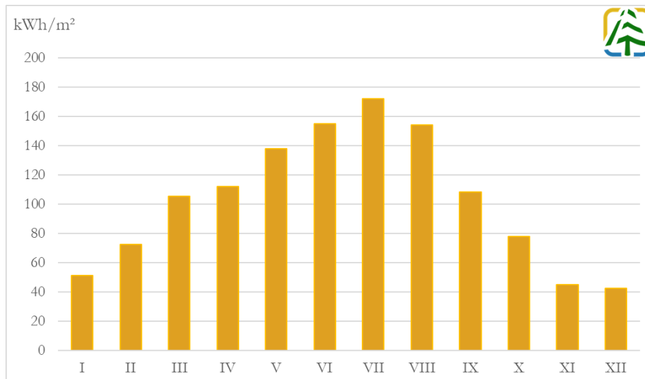
Slika 4.23 Godišnji hod izravnog normalnog sunčevog zračenja na području Hrvatske Dubice (Izvor: Global Solar Atlas)
