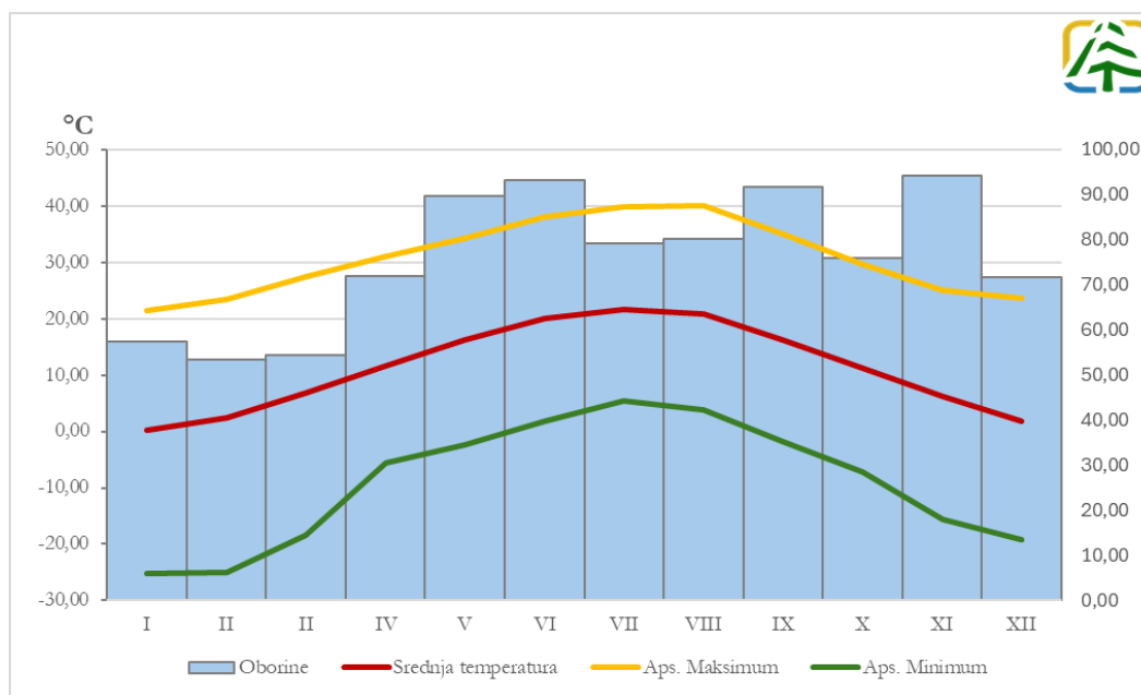
Slika 4.22 Srednje mjesečne količine oborine i temperature za meteorološku postaju Sisak u razdoblju 1949. -2023. (Izvor: DHMZ)
