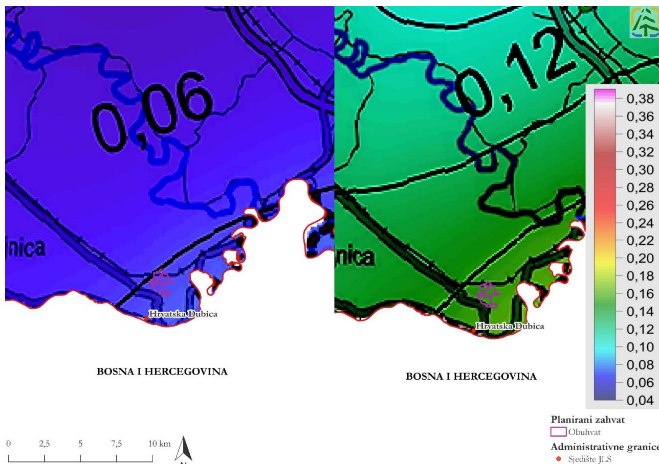
Slika 4.32 Karta horizontalnih vršnih ubrzanja tla tipa A s vjerojatnosti premašaja 10 % u 10 godina za povratno razdoblje 95 godina (lijevo) i poredbenih vršnih ubrzanja tla tipa A s vjerojatnosti premašaja 10 % u 50 godina za povratno razdoblje 475 godina (desno) izražena u jedinicama gravitacijskog ubrzanja (g) (Izvor: Idejno rješenje i Herak i dr., 2011)
