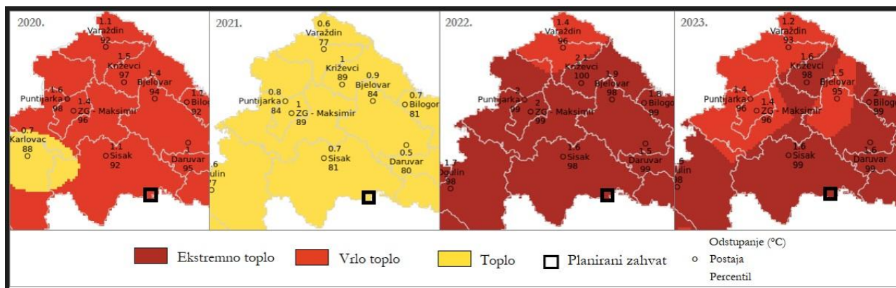
Slika 4.24 Odstupanje srednje temperature zraka u razdoblju 2020. – 2023. godine na širem području planiranog zahvata (Izvor: DHMZ)
