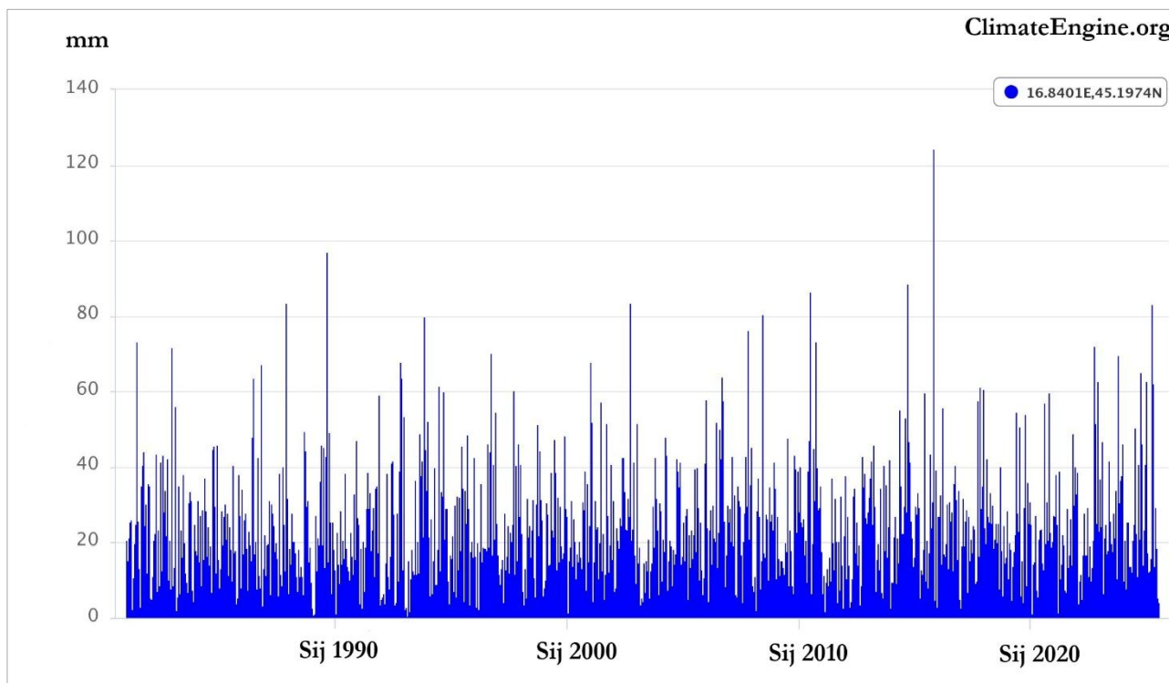
Slika 5.5 Prikaz količine oborina na području planiranog zahvata u razdoblju 01.01.1981. – 26.06.2025. (Izvor: Climate Engine )
